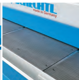
Auflagetisch mit Maßeinteilung und ausziehbare Blechauflage
